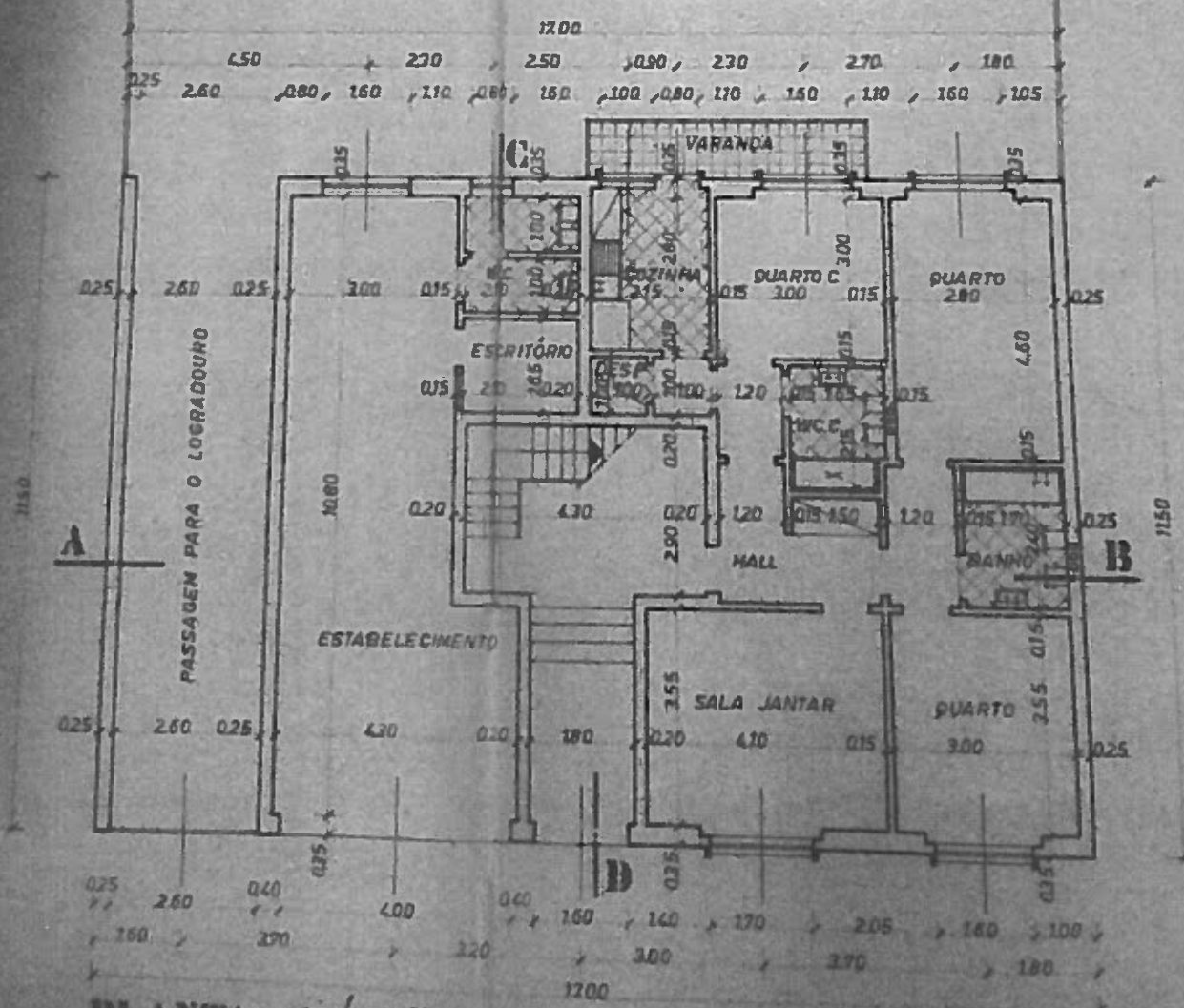
PLANTA R/CHÃO
